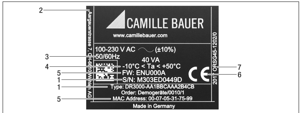
1 Typenschild des Gerätes (beispielhaft)
