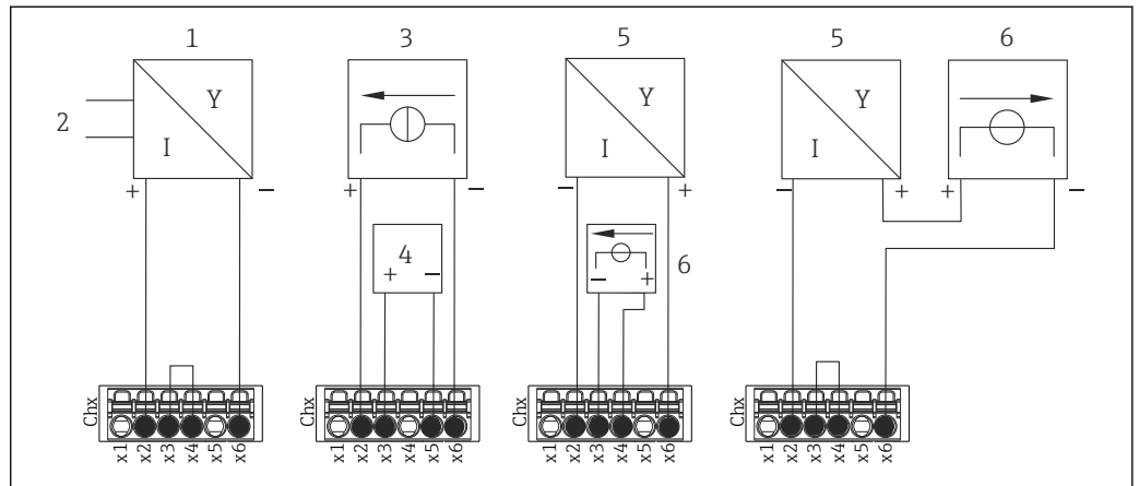
8 Anschlussbeispiel HART®-Eingänge in einer Punkt-zu-Punkt-Verbindung
