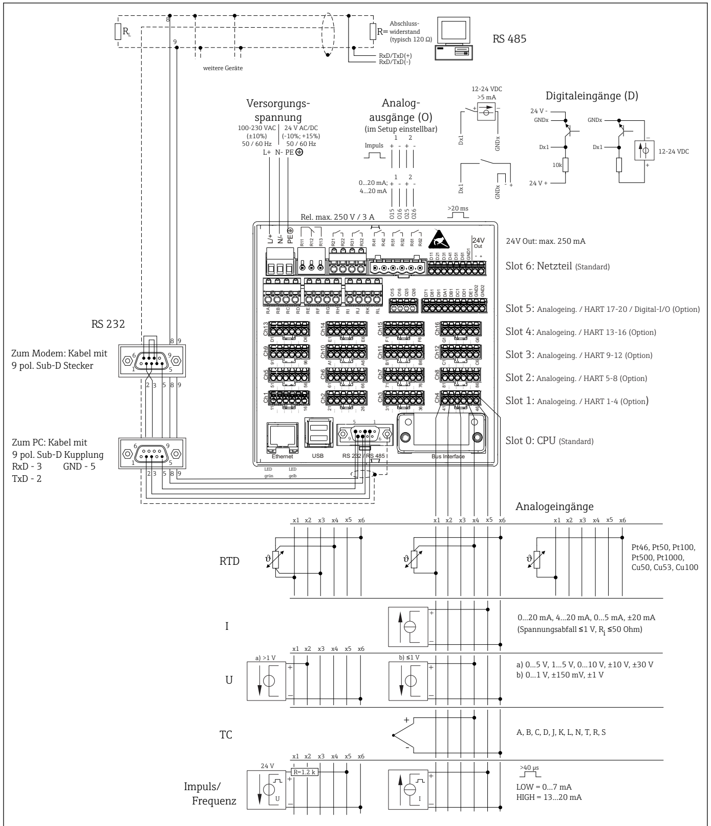
17 Anschlussbeispiele der HART®-Eingänge (optional) siehe Betriebsanleitung → 23
