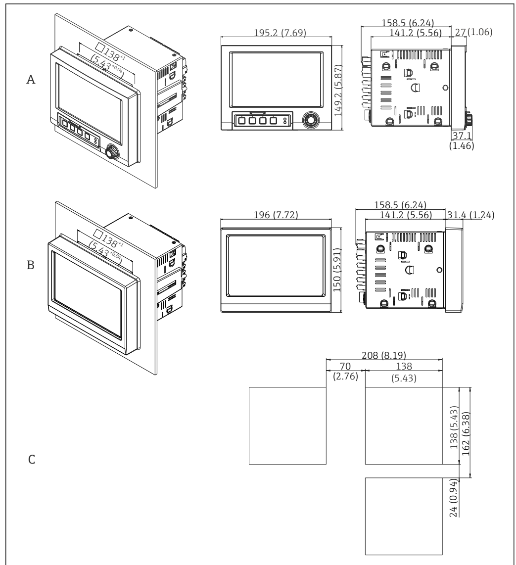
18 Schalttafeleinbau und Maße in mm (in).
