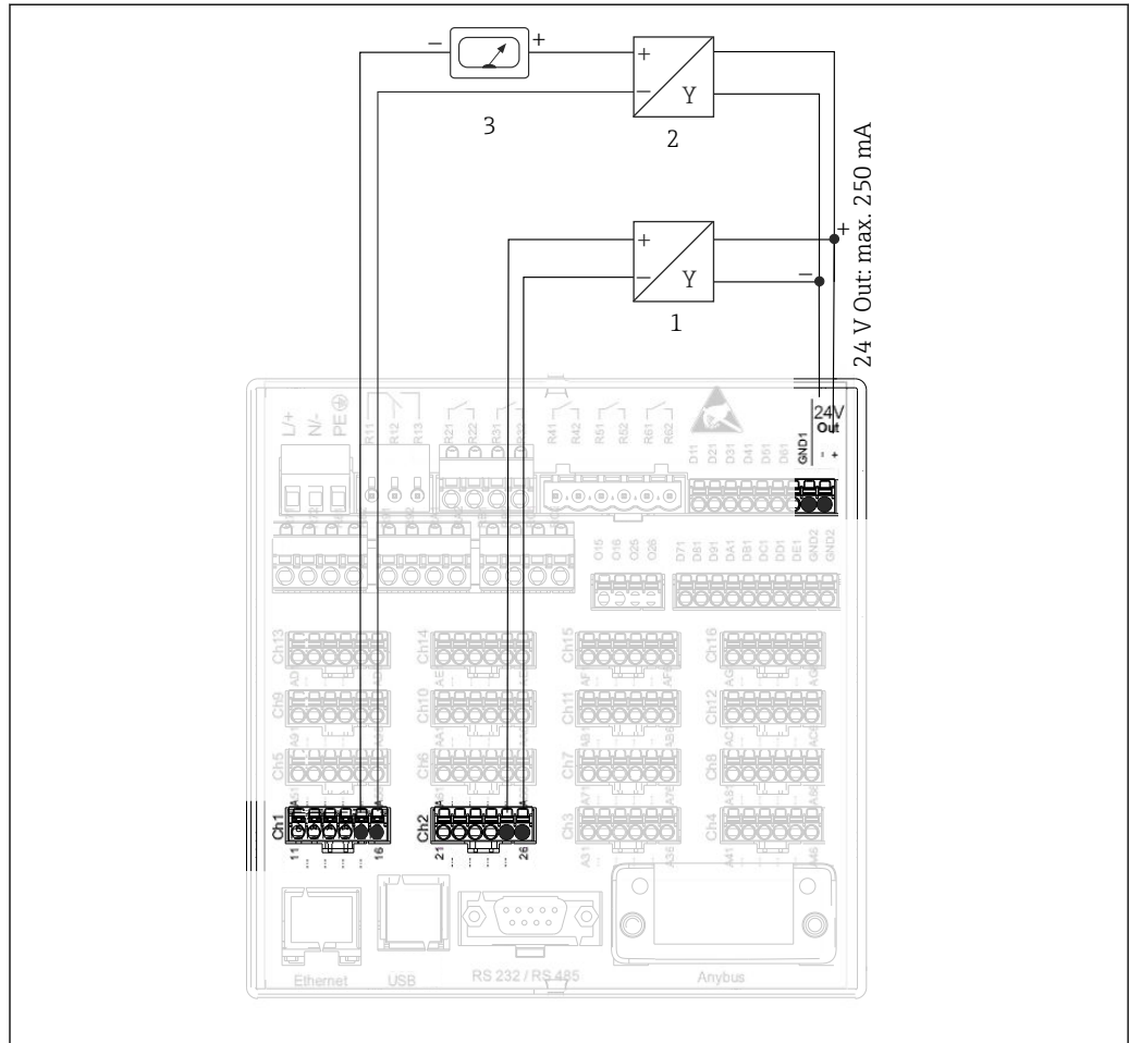
7 Anschluss des Hilfsspannungsausgangs bei Verwendung als Messumformerspeisung (MUS) für 4-Leiter-Sensoren im Strommessbereich
