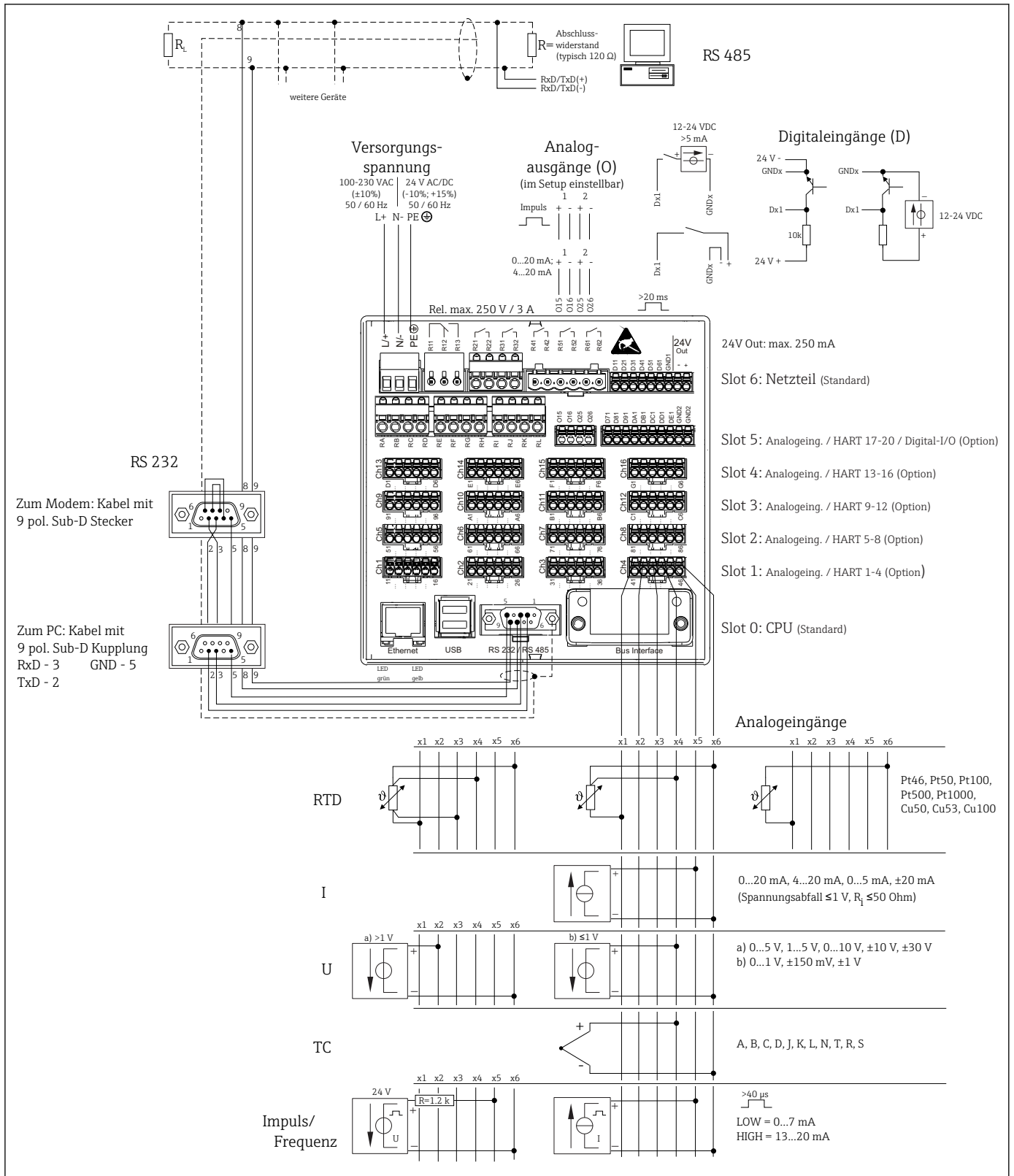
5 Anschlussbeispiele der HART®-Eingänge (optional) siehe Betriebsanleitung → 23
