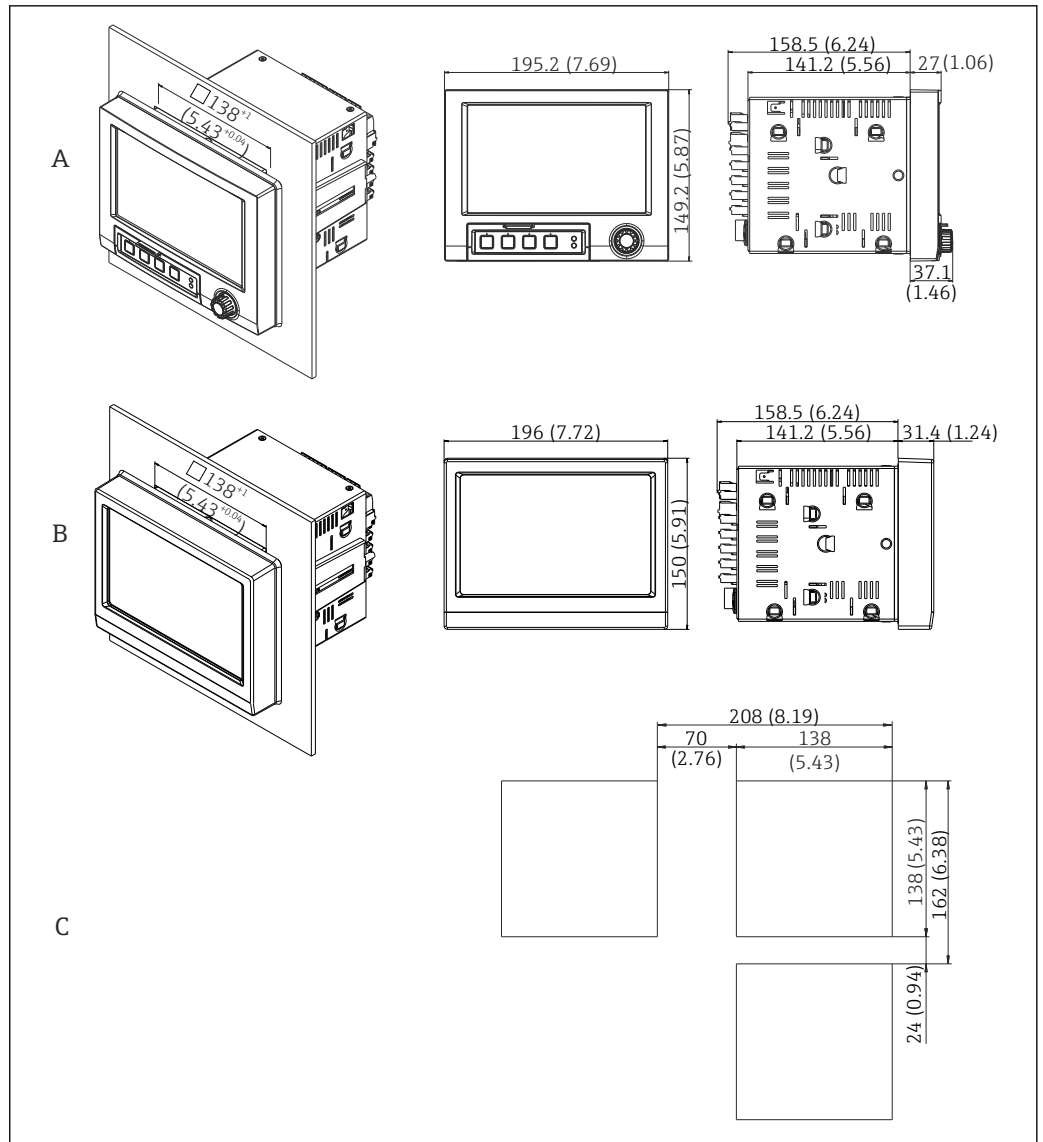
2 Schalttafelausschnitt und Maße in mm (in).
