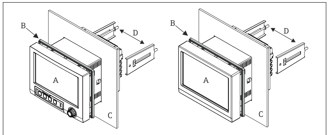
3 Schalttafeleinbau
