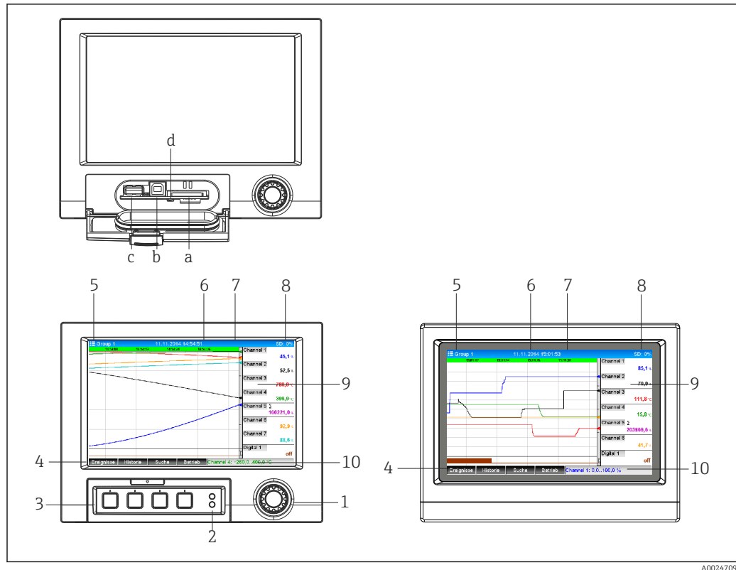
12 Gerätefront (links: Version mit Navigator und Frontschnittstellen; rechts: Version mit Edelstahlfront und Touchscreen)
