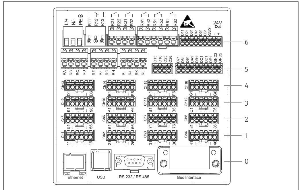
16 Anschlüsse Geräterückseite
