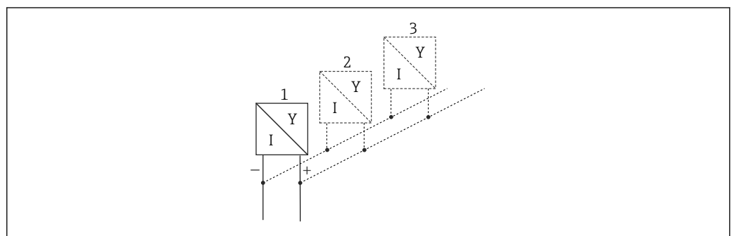
9 Anschlussbeispiel HART®-Eingänge in einer Multidrop-Verbindung
