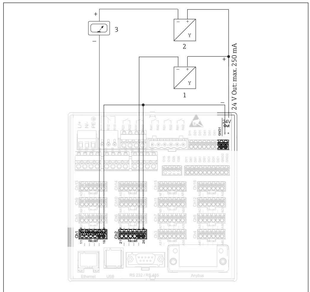
6 Anschluss des Hilfsspannungsausgangs bei Verwendung als Messumformerspeisung (MUS) für 2-Leiter-Sensoren im Strommessbereich
